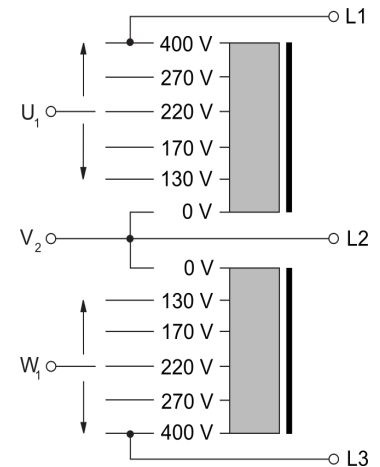
ATT connection diagram
